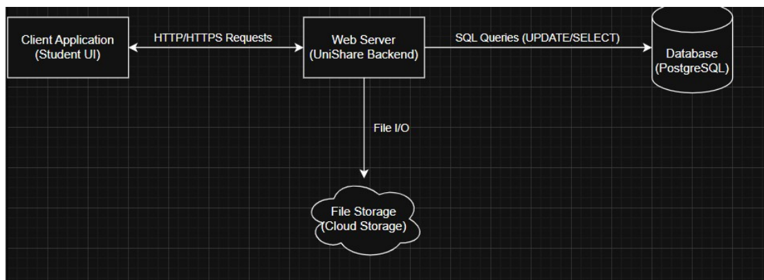
Рисунок 1 - Архітектура UniShare
